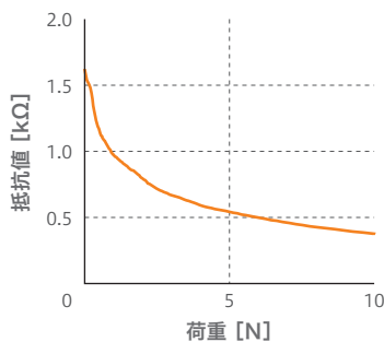
荷重 - 抵抗値 特性図
