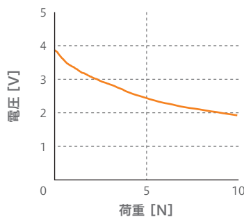
荷重 - 電圧 特性図
